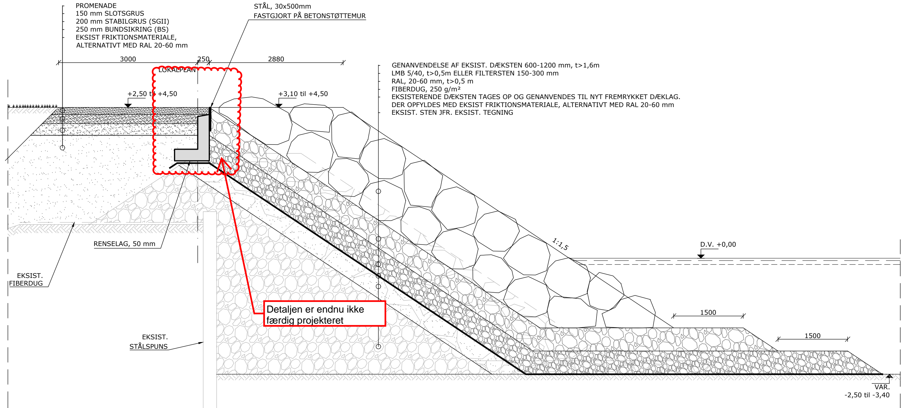
Tværsnit A-A, ST. -22,55 til ST. 46,00
